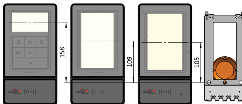
DETAIL 1 - Maßstab 1 : 4
