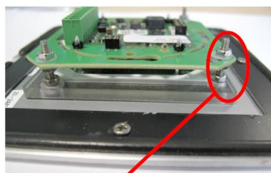
Ansicht Rückseite (Abstand Leseinheit – Blende)
