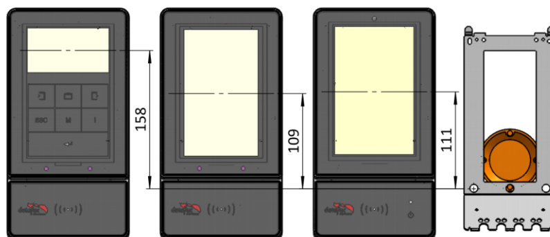
DETAIL 1 - Maßstab 1 : 4
