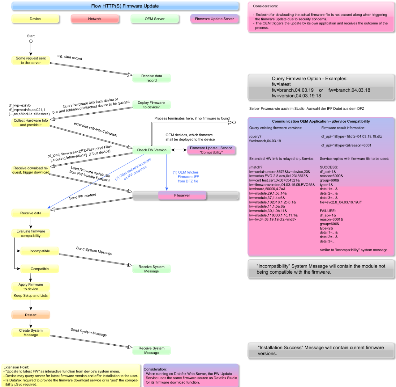
Diagramm zum Ablauf des Firmware-Updates
