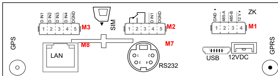
Steckerleiste des EVO 2.8 Pure V4
